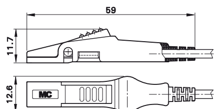
Ø 1,5 mm-Stecker, vergoldet, PA-Isolation, montiert Ø 1,5 mm plug, gold-plated, PA insulation, assembled
