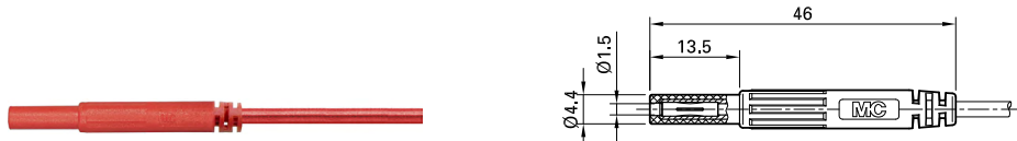
Ø 1,5 mm-Buchse, vergoldet, TPE-Isolation, umspritzt Ø 1,5 mm socket, gold-plated, TPE insulation, moulded
