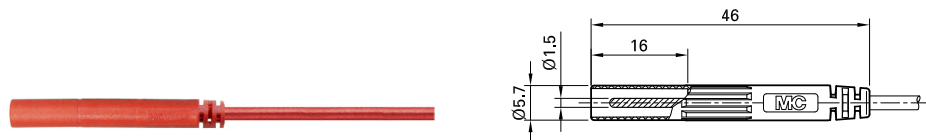
Ø 1,5 mm-Stecker, vergoldet, TPE-Isolation, umspritzt Ø 1,5 mm plug, gold-plated, TPE insulation, moulded
